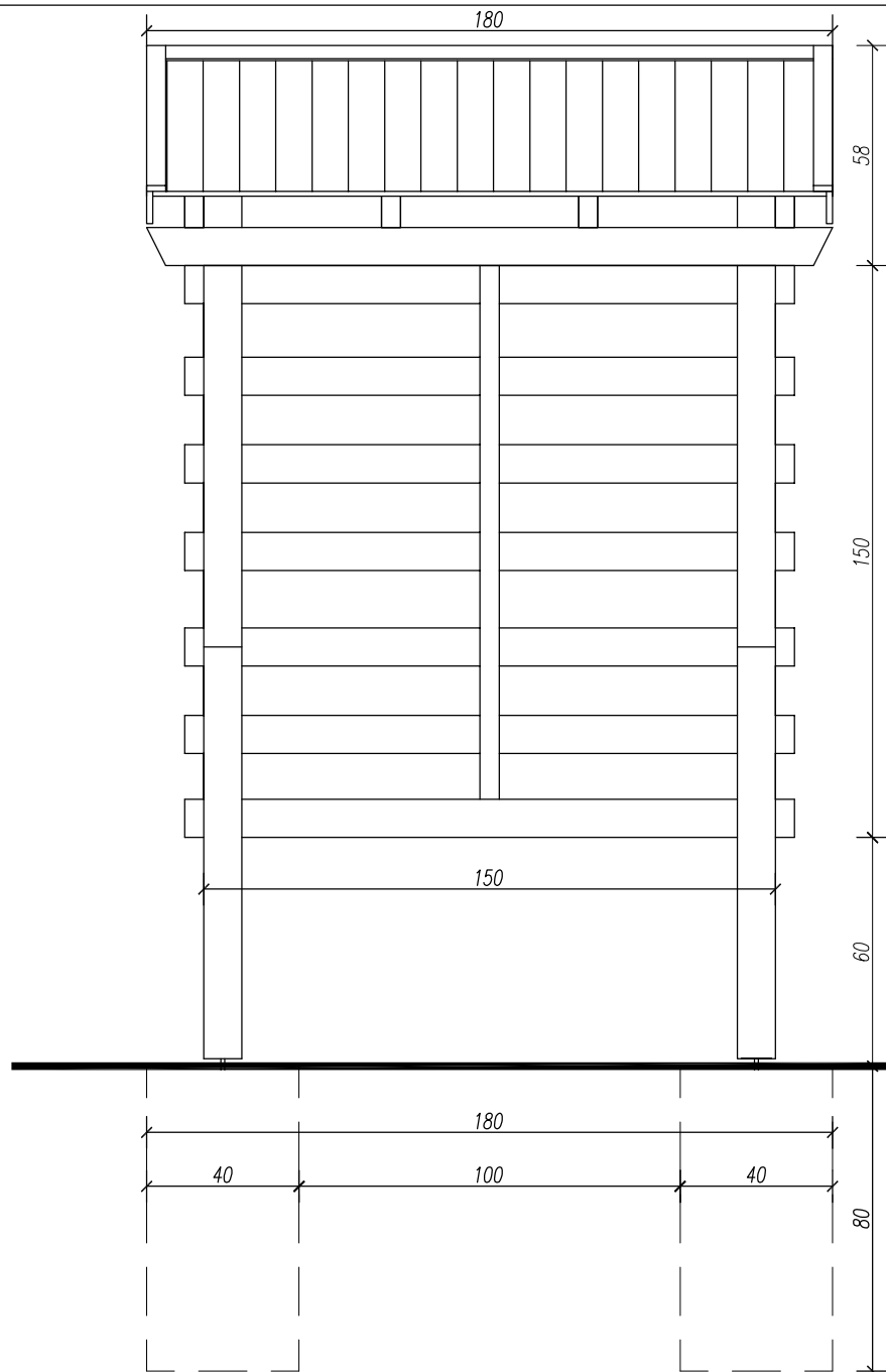
WIDOK - TYŁ
